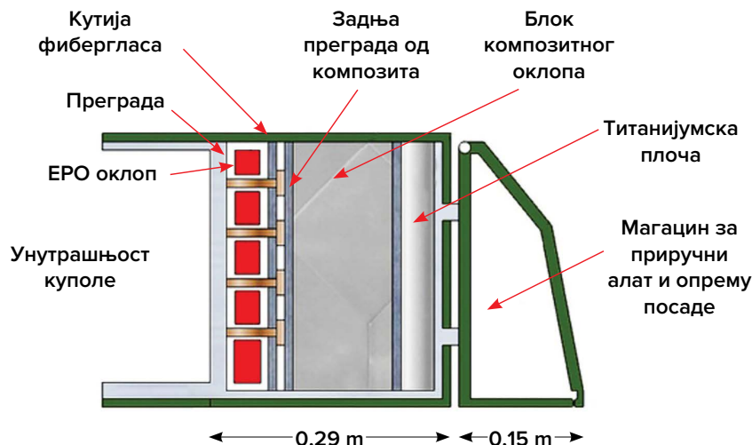
Пресек бочног оклопа куполе Леклерк XXI (3. серија)
