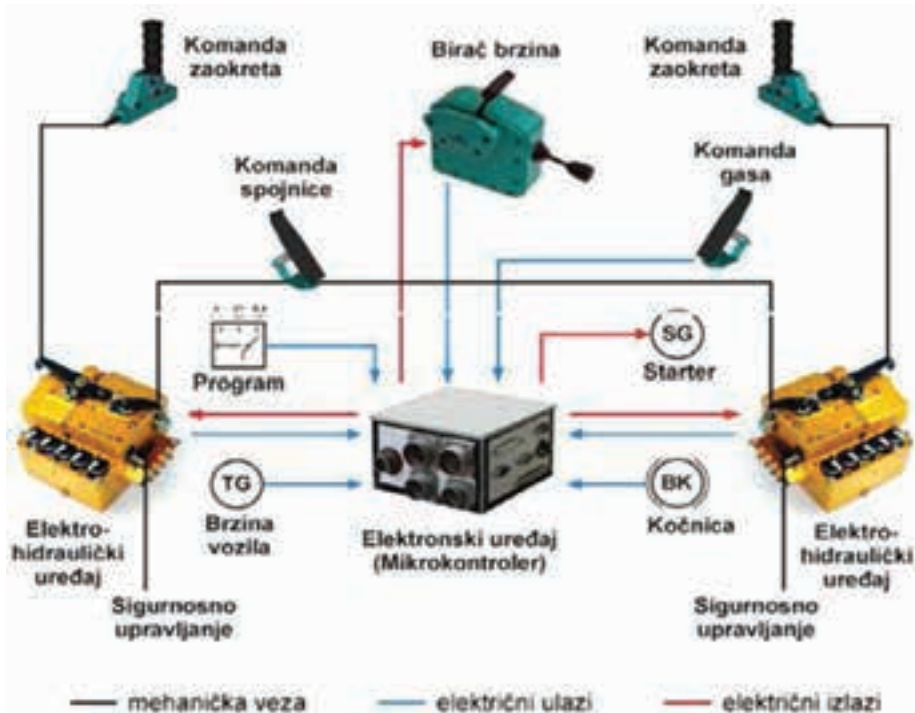
Електрохидраулични систем за аутоматско управљање трансмисијом са два бочна планетарна мењача
